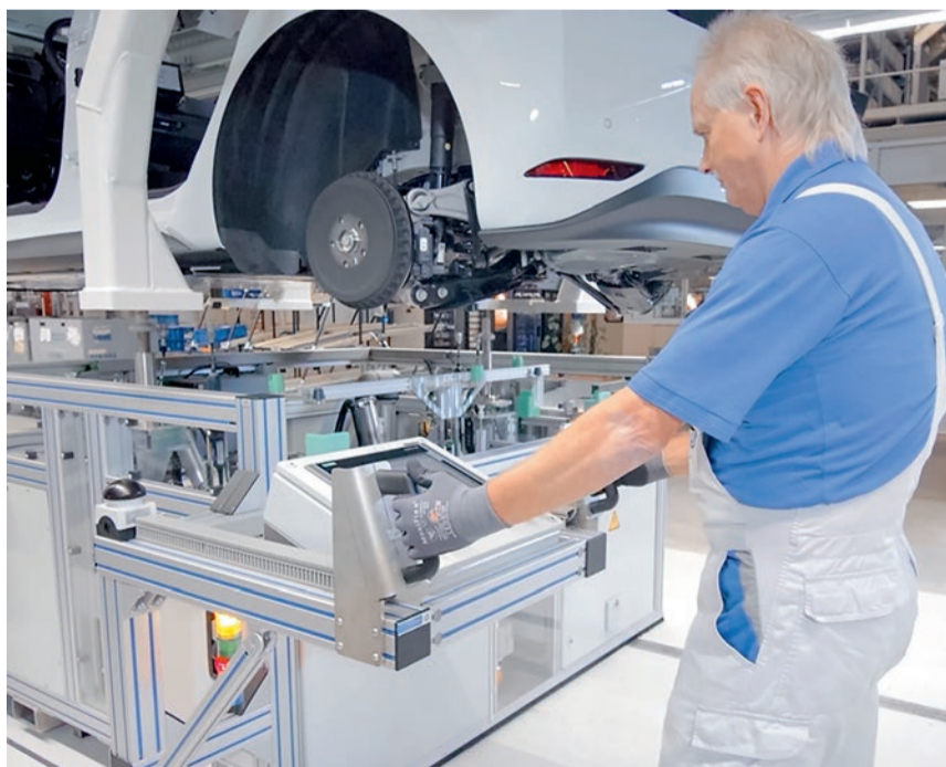
Hilfsmittel für die Mitarbeiter: Der Montagewagen verbessert die Ergonomie am Arbeitsplatz.
